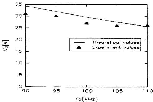
그림 10. 동작주파수 vs. 출력전압의 실험특성
