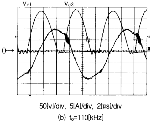
그림 8. V_{c1} 과 V_{c2} , I_1 의 실험파형
