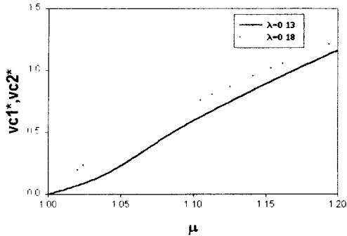
그림 3. 정규화 주파수 vs. V_{o1}^* , V_{o2}^* 의 이론특성
