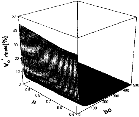
그림 6. 정규화 캐패시터비 vs. 출력전압 리플의 이론특성
