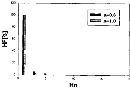
그림 7. 고조파 함유율의 이론특성
