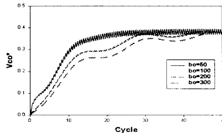
그림 4. 출력전압의 기동과도 이론특성( V_{co} )
