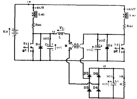
그림 1. ZVS를 이용한 Push Pull형 고주파 DC-DC 컨버터
